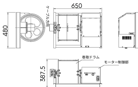
巻き取りドラム JD-HMW1
